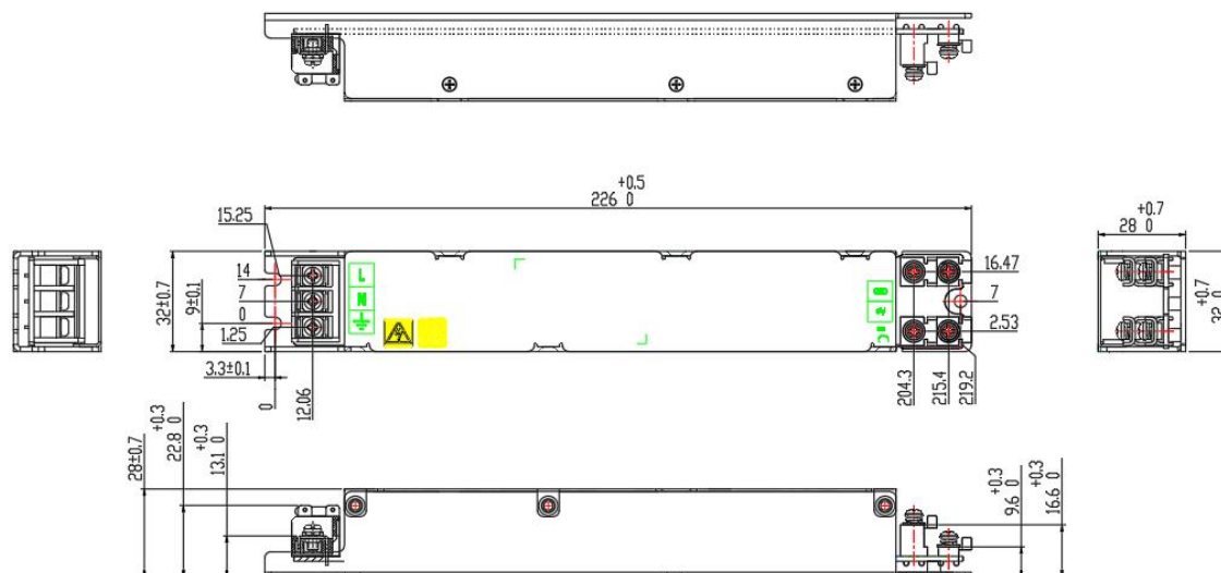
外形尺寸及安装孔——端子坐标
